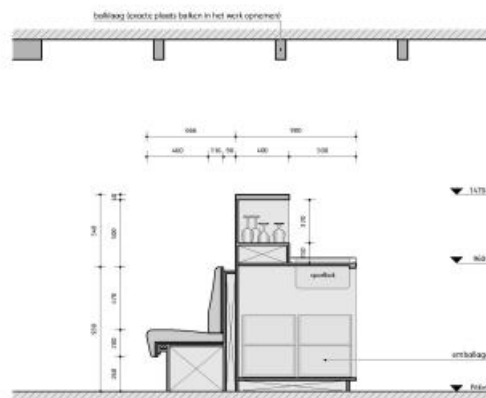
Principedoorssnede A-A 1:20 bar / bar
