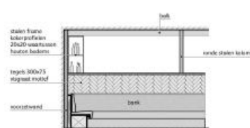
Aanzicht 2 1:50 bar / zijkant bar
